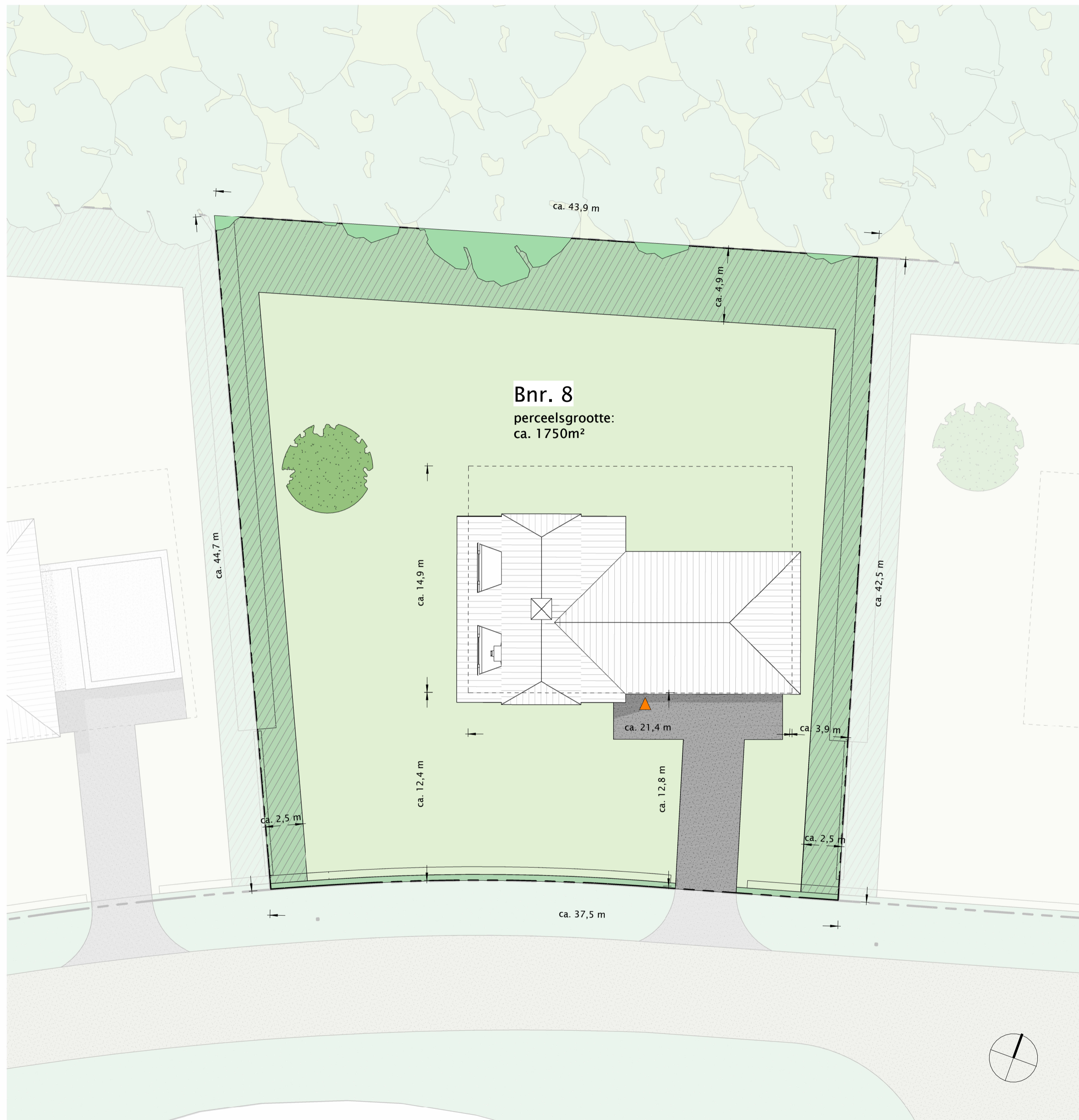
kavel bouwnummer 8 1 : 200
